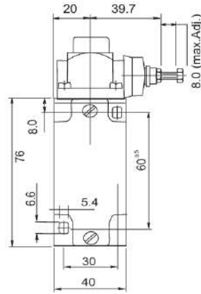
KLSPBA
