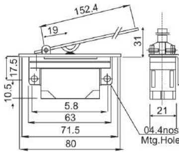
KLSILR1 KLSILR2
