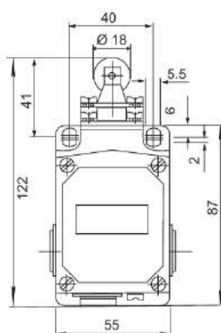
KLPRSO KLPRO
