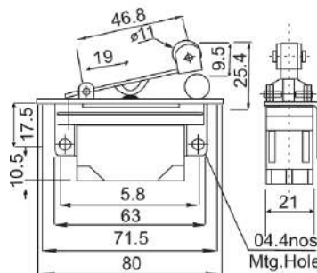
KLRL1 KLRL2
