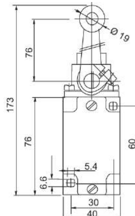
KLSL2
